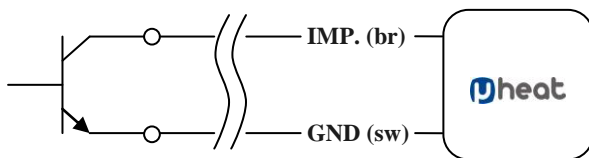
Impulseingangsbeschaltung mit bipolar. Transistor
