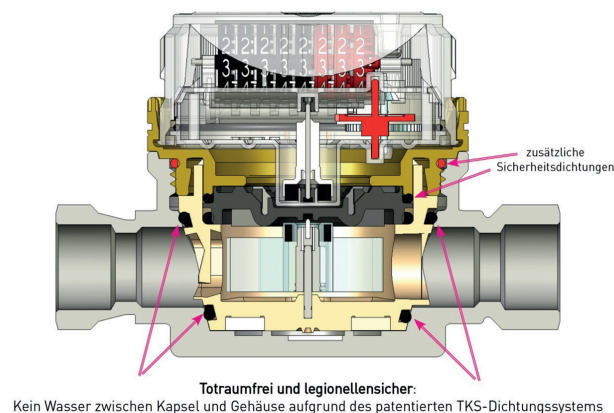
Patentiertes DELTAMESS-TKS-Kapselsystem
